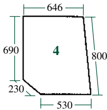
21/4034-1 (D7043, 04316723) Porte (Haut droit) Door (Upper RH)
