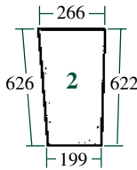
21/4016-2 (D7041, 04316654) Avant (Bas droit) Front (Lower RH)
