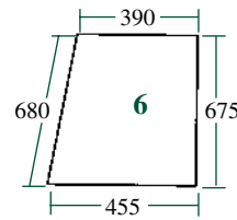
21/4041-5 (D7048/F) Latérale (Fixe, gauche ou droit) Side (Fixed, LH or RH)
