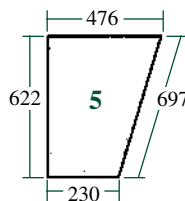
21/4032-1 (D6769, 04316720) Porte (Bas gauche) Door (Lower LH)
