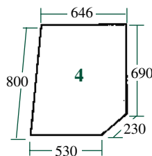
21/4035-1 (D7044, 04316724) Porte (Haut gauche) Door (Upper LH)
