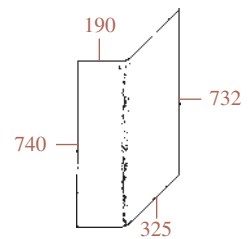
23/4086-3 (5154093) Arrière coin droit - verte Rear quarter RH - green
