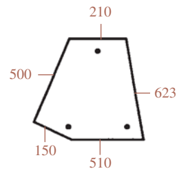
23/4065-4 (D9023, 5130895) Latérale gauche - verte 3 trous Side LH - green 3 holes
